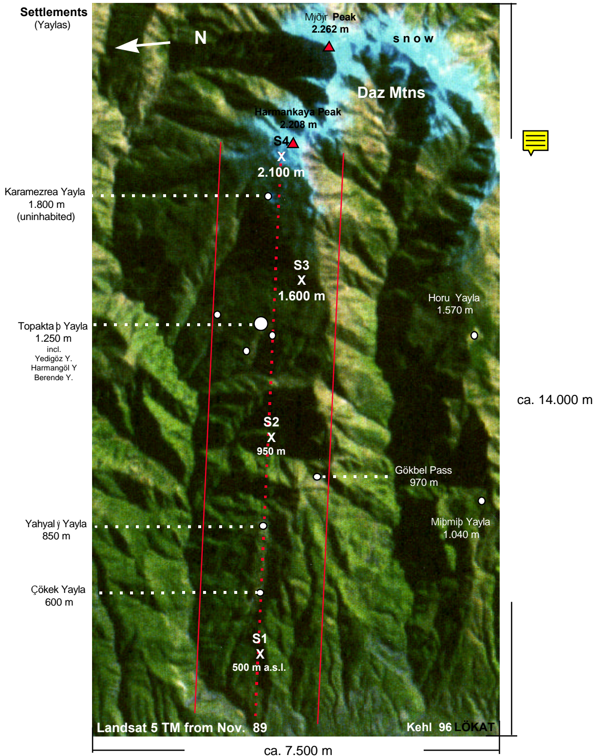
Foto Nr. 11-3: Geometrisch korrigiertes Farbkompositenbild aus Landsat 5 TM-Daten von der Westabdachung des Amanus oberhalb von Dörtiyol (SE-Türkei) vom N o v e m b e r 1989 mit dem UG LÖKAT (gleicher Ausschnitt wie Foto Nr. 11-2). Gipfelgruppe der Daz Dađları ist schneebedeckt. Der (Tages)Zeitpunkt beider Aufnahme ist gleich. Zu beachten sind daher die unterschiedlichen Schattenbilder, die nahezu laubfreie mittel- bis hochmontane Zone und die sich bis in den Buchenwald erstreckende Schneebedeckung. Für Yedigözü Yayla (1.050 m ü. NN) wurden von Yaylabauern maximale Schneehöhen > 70 cm mitgeteilt.
